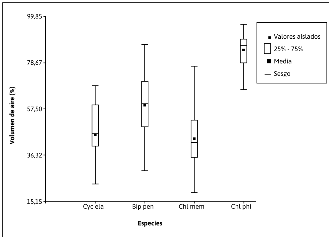
Figura 4. Gráfico de caja (box-plot) para el volumen de aire de las semillas de 4 orquídeas terrestres. Cyc ela: Cyclopogon elatus ; Bip pen: Bipinnula pennicillata ; Chl mem: Chloraea membranacea y Chl phi: Chloraea philippii
