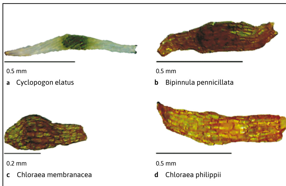
Figura 1. Microfotografías de las semillas de orquídeas terrestres (a, b, c y d), donde se observa claramente la posición y tamaño del embrión ocupando la parte central y de color más oscuro de la imagen y la estructura reticulada de la testa en b, c y d
